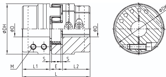
ROTEX® 38 - 90
