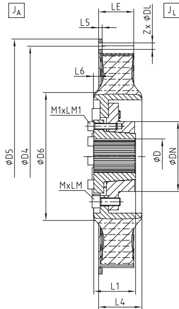
Type AKC
