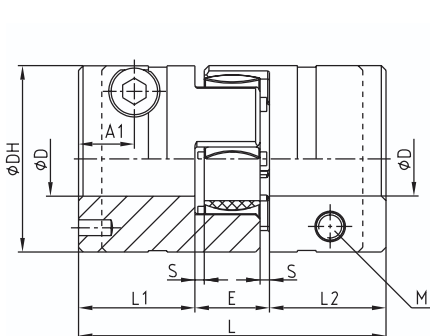
ROTEX® 19 - 28
