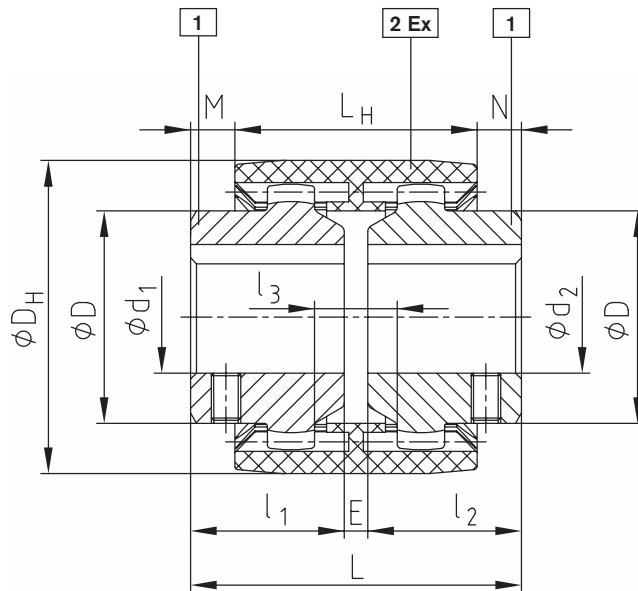
Type M...C
