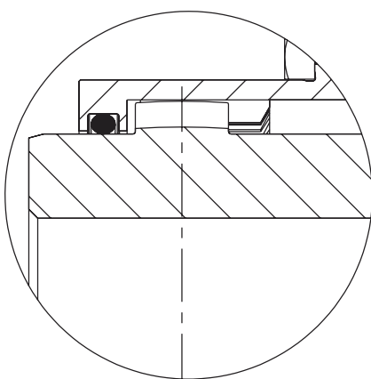
Type FR
