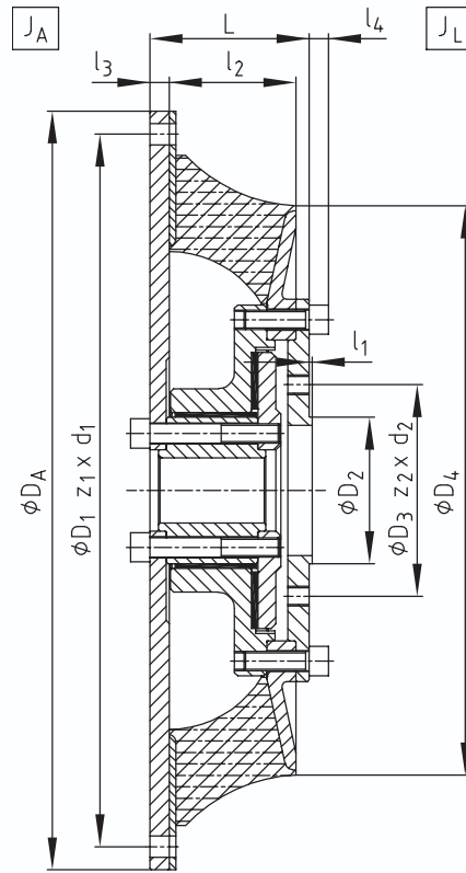
Type HEG1
