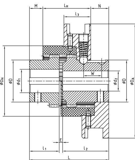
BoWex® SD2
