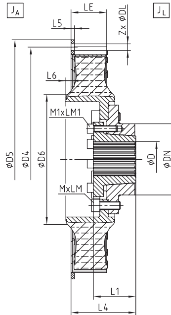
Type ALC
