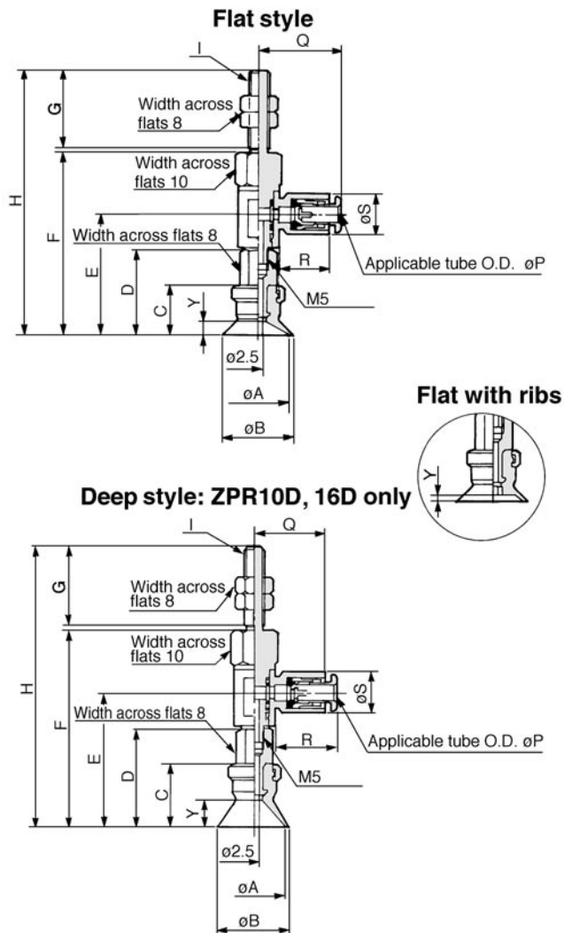
Pad Diameters ø10, ø13, ø16
