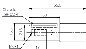
Eje forma R / Shaft form R
