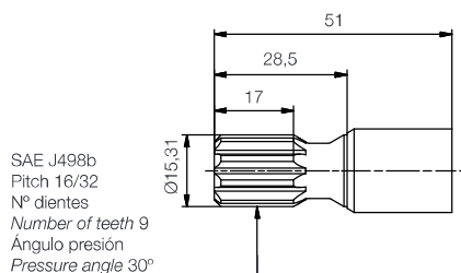
Eje forma G / Shaft form G
