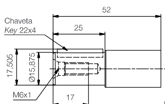
Eje forma H / Shaft form H
