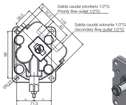
Bomba giro izquierda Counterclockwise rotation pump
