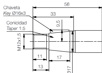
Eje forma J / Shaft form J
