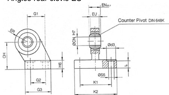
Angles rear clevis ES
