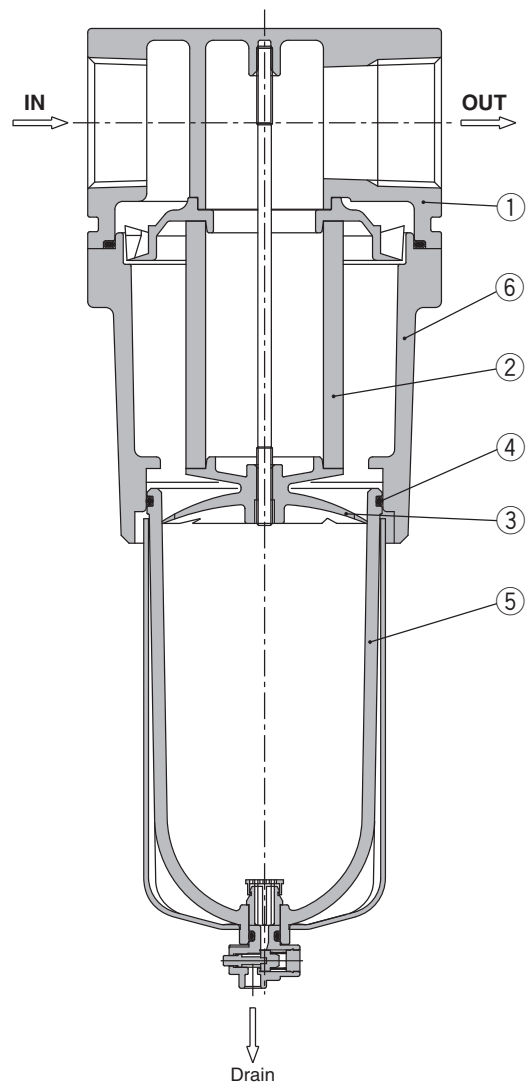
AF50, AF60
