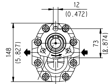
Flange T1
