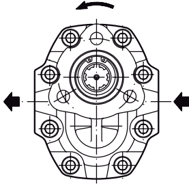
ANT-CLOCK ROTATION
