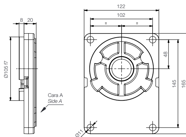
Tapa tipo 23 / Front flange type 23
